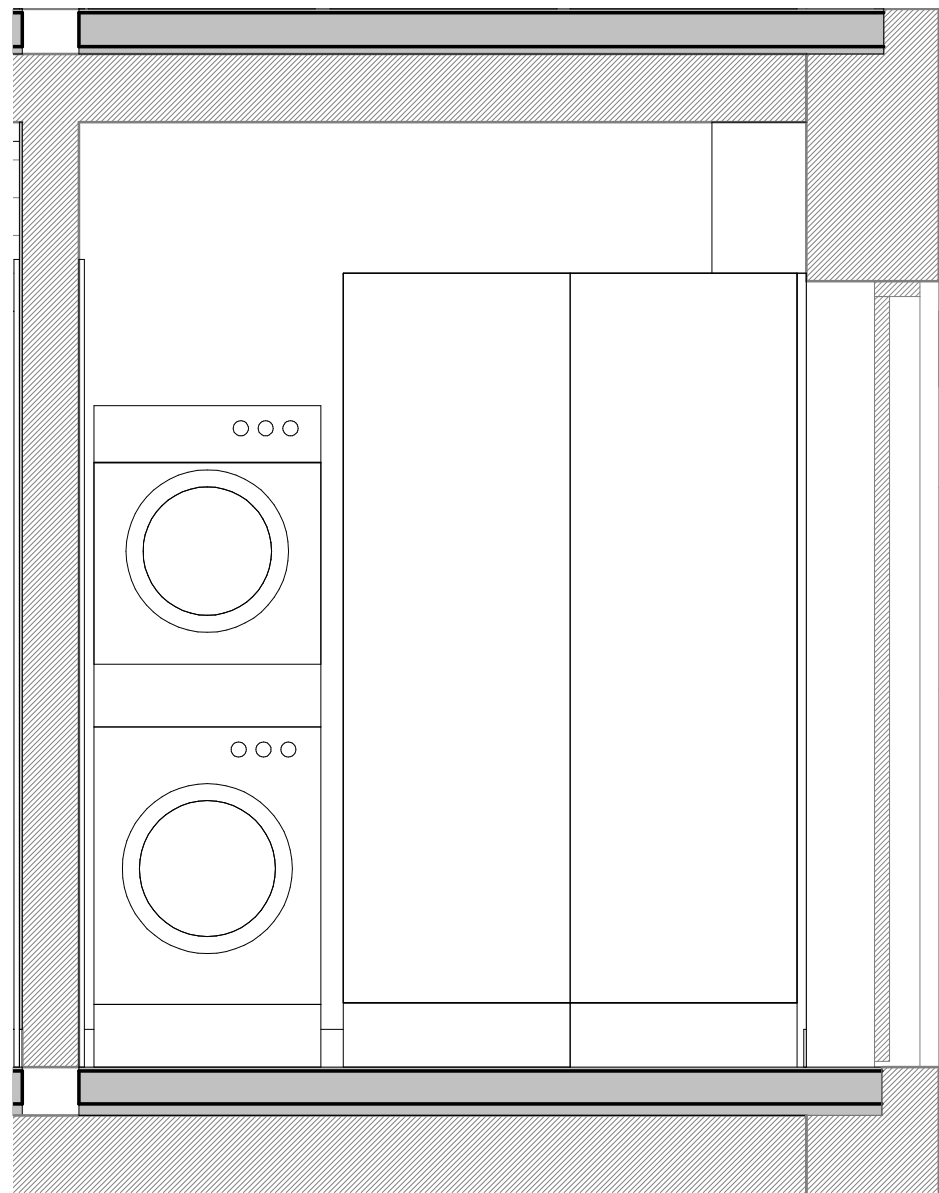
Entré Opstalt 5 Type CD | 1 : 20
