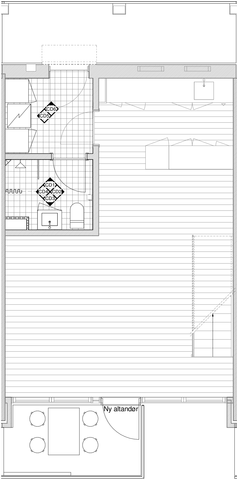
Blok 7, 1. sal Type D | 1 : 50
