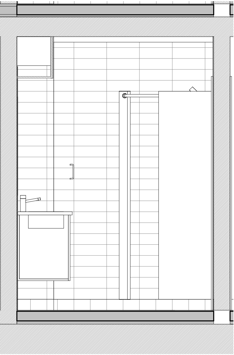
Badeværelses Opstalt 4 Type CD | 1 : 20
