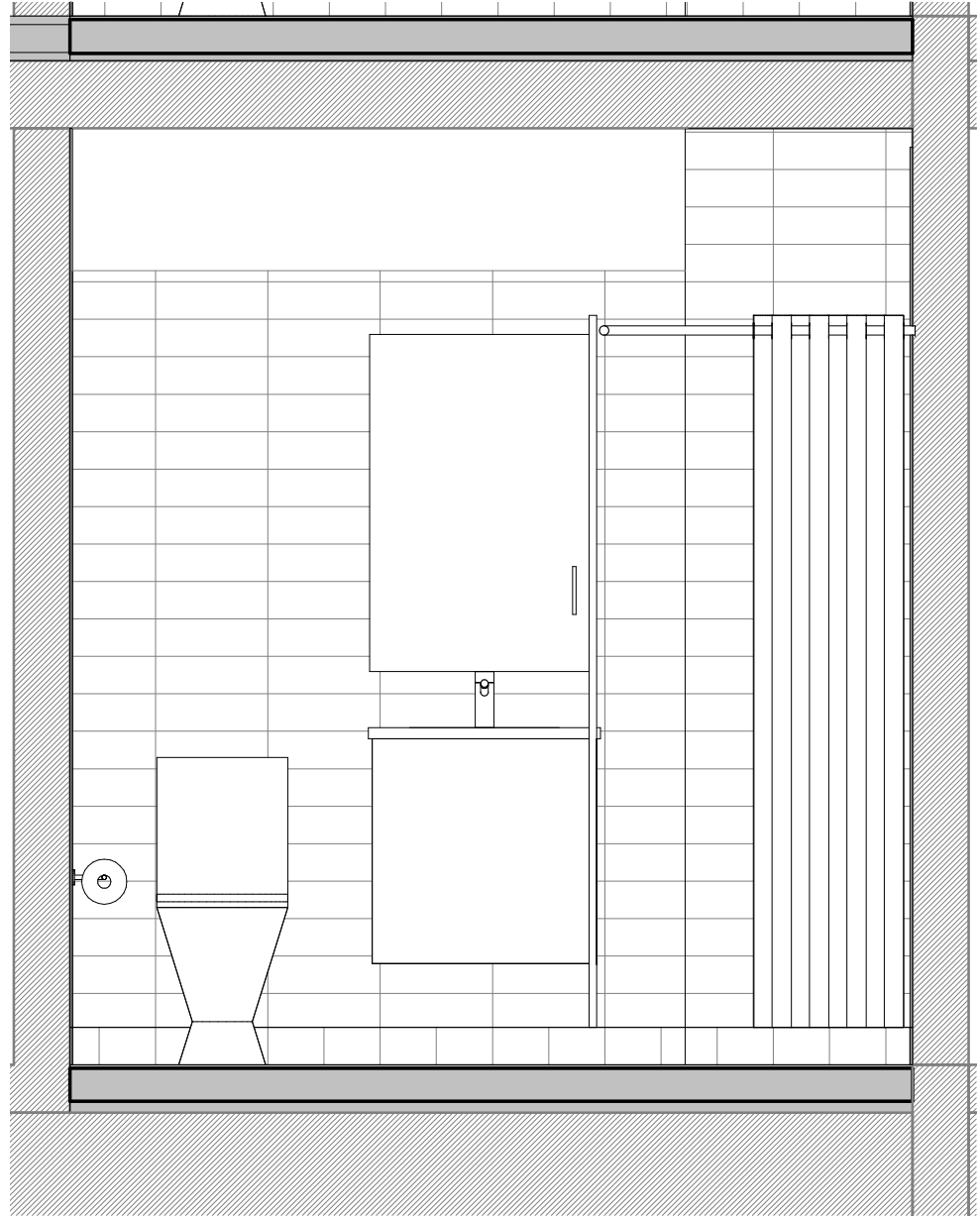
Badeværelses Opstalt 3 Type CD | 1 : 20
