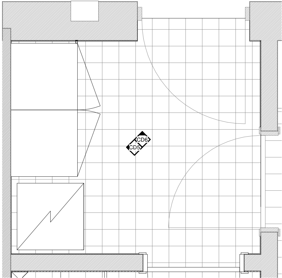
Blok 7, Entré Type CD | 1 : 20
