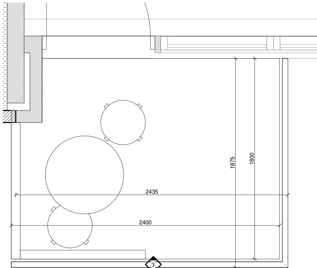
Planudsnit Lille Altan | 1 : 20
