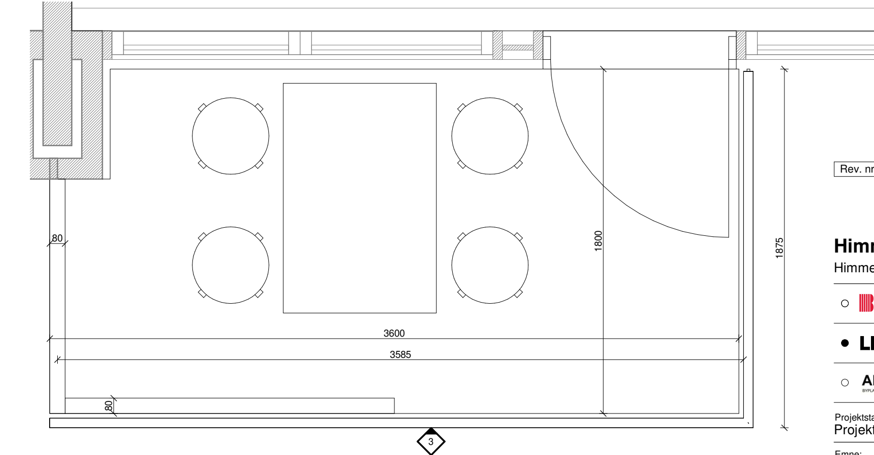
Planudsnit Stor Altan | 1 : 20
