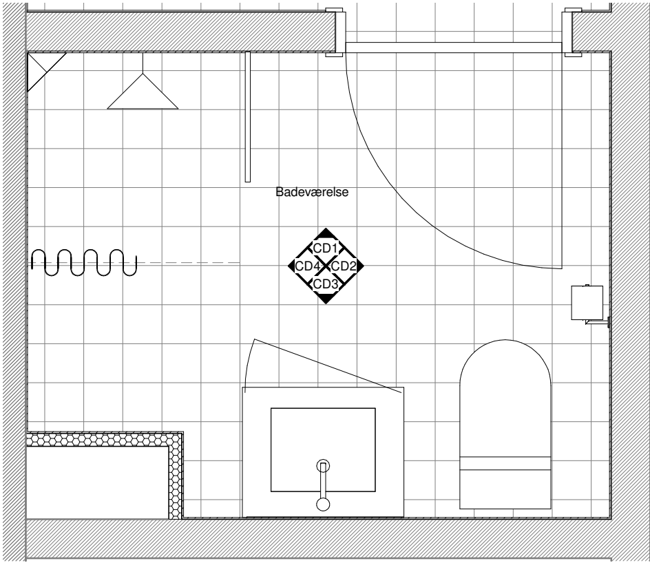
Blok 7, Badeværelse Type CD | 1 : 20
