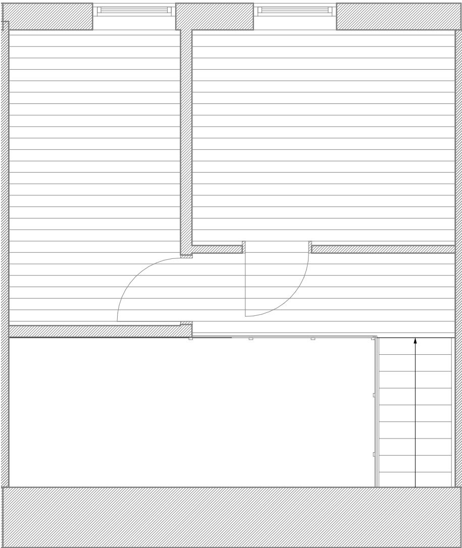
Blok 7, 2. sal Type D | 1 : 50
