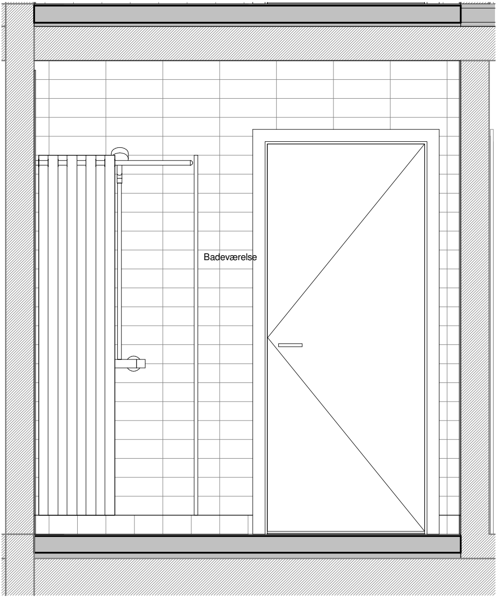
Badeværelses Opstalt 1 Type CD | 1 : 20
