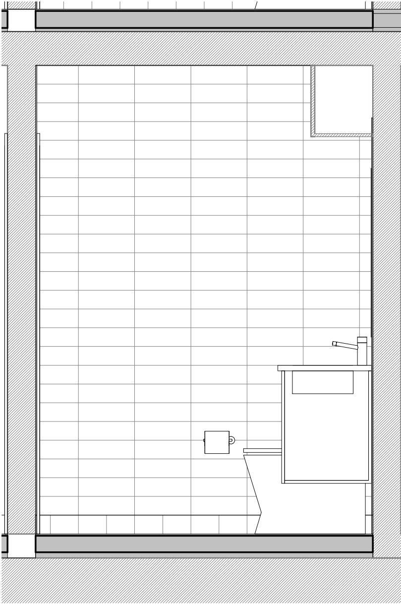
Badeværelses Opstalt 2 Type CD | 1 : 20
