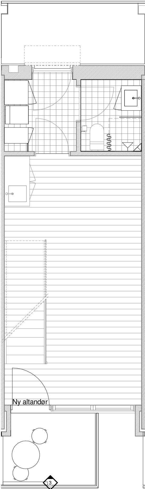
Blok 7, 1. sal Type B | 1 : 50
